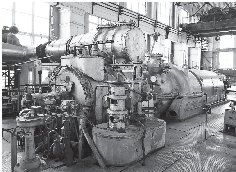
Турбина Ленинградского механического завода им. И.В. Сталина, 1937 г. Самарская ГРЭС
