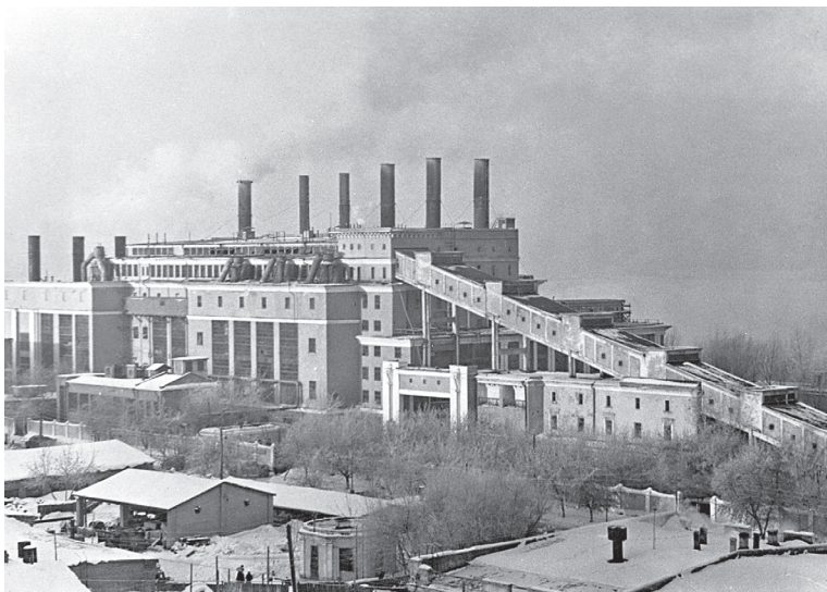
Производственные корпуса Куйбышевской ГРЭС после реконструкции 1937–1941 годов
