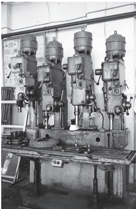
Трофейный сверлильный станок «Stenzel»
